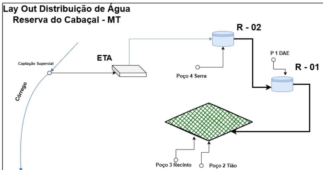
Figura 3 - Layout Concepção de Abastecimento de Água da Cidade de Reserva do Cabaçal-MT - AGERR Pantanal
