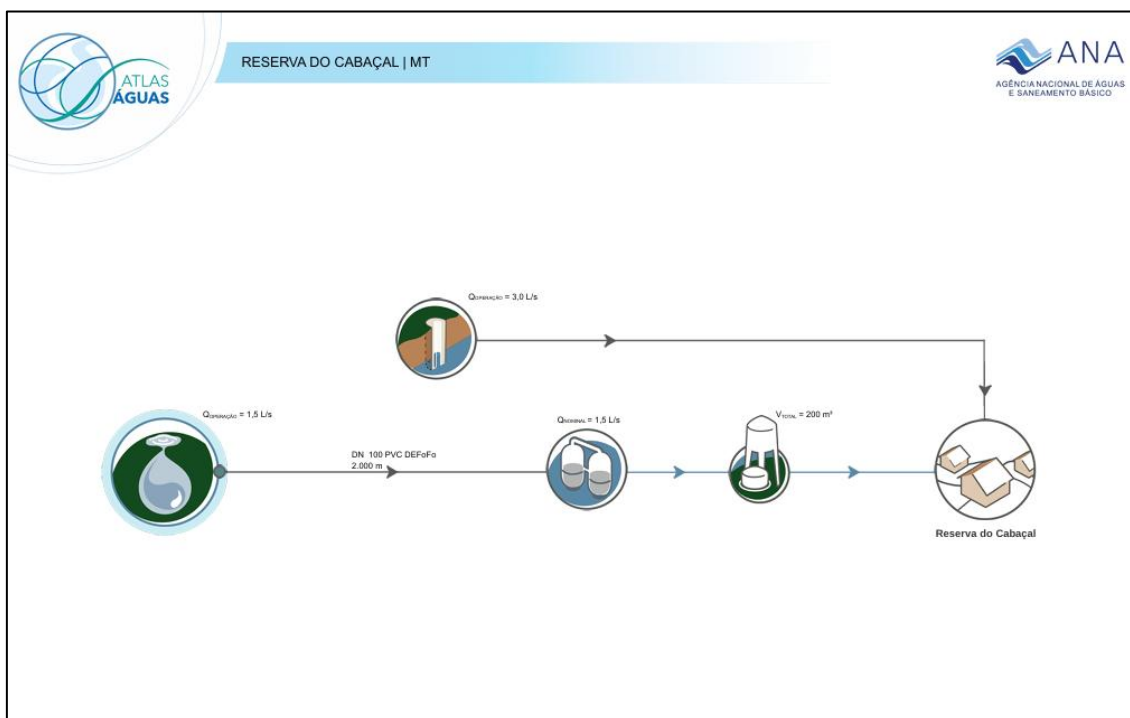
Figura 2 – Desenho ilustrativo do SAA de Reserva do Cabaçal - MT
